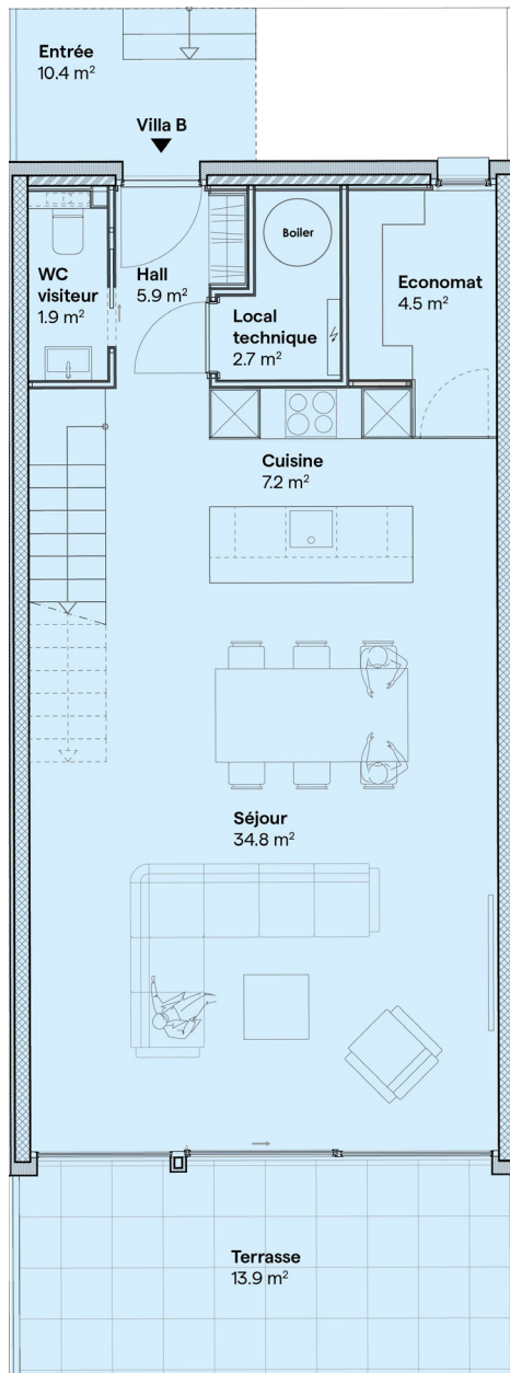
REZ - DE - CHAUSÉE
